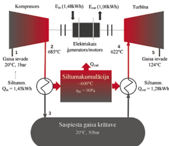
5. attēls. Adiabātiskas saspiesta gaisa enerģijas akumulācijas stacijas darbības shēma
